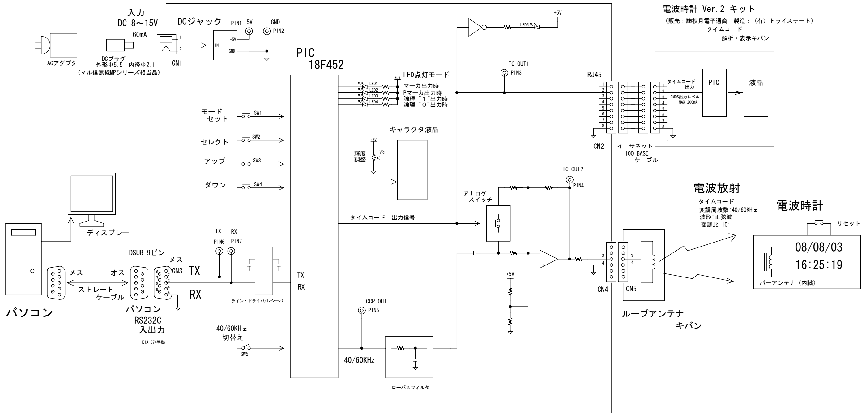
JJY日本標準時シミュレーター キット 周辺部品接続図
